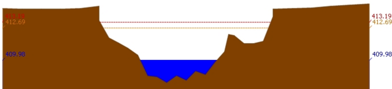
สถานี 070110T แม่น้ำวังที่ อ.วังเหนือ ต.วังเหนือ อ.วังเหนือ จ.ลำปาง ระดับน้ำ 409.98 ม.รทก.
