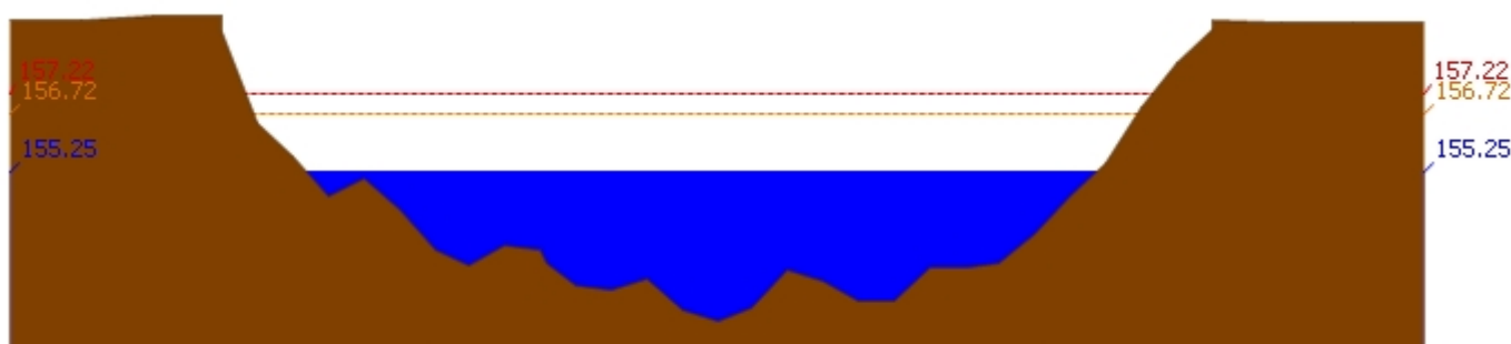
สถานี 070117T แม่น้ำวังที่เทศบาลตำบลแม่ป๋อ ต.แม่ป๋อ อ.แม่พริก จ.ลำปาง ระดับน้ำ 155.25 ม.รทก.
