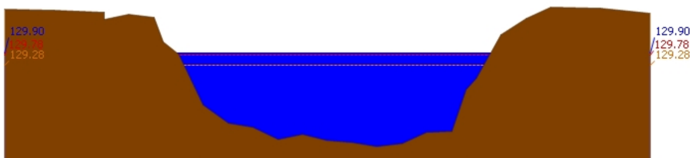
สถานี 070118T แม่น้ำวังที่บ้านแม่สลิด ต.แม่สลิด อ.บ้านตาก จ.ตาก ระดับน้ำ 129.90 ม.รทก.
