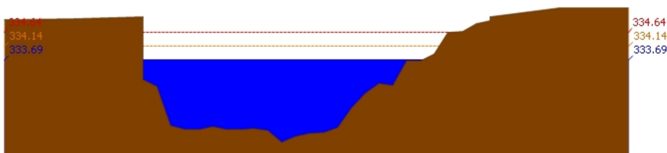
สถานี 070304T น้ำแม่สอยที่บ้านหนองกอก ต.แม่สวก อ.แจ้ห่ม จ.ลำปาง ระดับน้ำ 333.69 ม.รทก.
