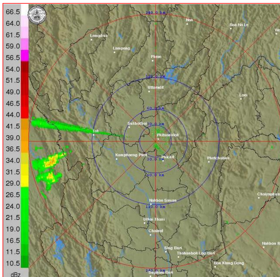
ภาพเรดาร์ตรวจอากาศ “พิษณุโลก” ณ วันที่ 2 กรกฎาคม 2561 (ที่มา : กรมอุตุนิยมวิทยา)
