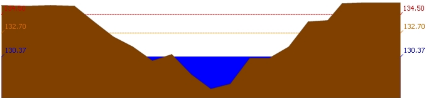
สถานี 120111T แม่น้ำป่าสักที่บ้านจางวาง ต.ลานบัว อ.หล่มสัก จ.เพชรบูรณ์ ระดับน้ำ 130.37 ม.รทก.
