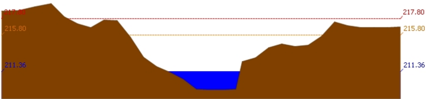
สถานี 120205T แม่น้ำป่าสักที่บ้านอู่กะทาด ต.ศิลา อ.หล่มเก่า จ.เพชรบูรณ์ ระดับน้ำ 211.36 ม.รทก.
