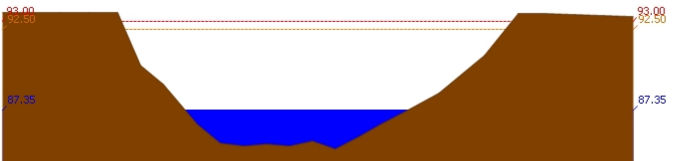
สถานี 120110T แม่น้ำป่าสักที่บ้านวังโบสถ์ ต.วังโบสถ์ อ.หนองไผ่ จ.เพชรบูรณ์ ระดับน้ำ 87.35 ม.รทก.
