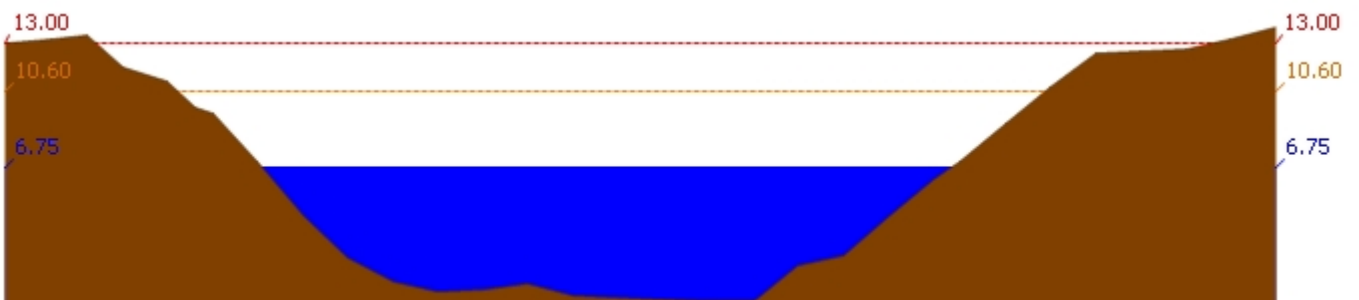
สถานี 120106T แม่น้ำป่าสักที่ อ.เสนาห์ ต.ศาลาวิไทย อ.เสนาห์ จ.สระบุรี ระดับน้ำ 6.75 ม.รทก.
