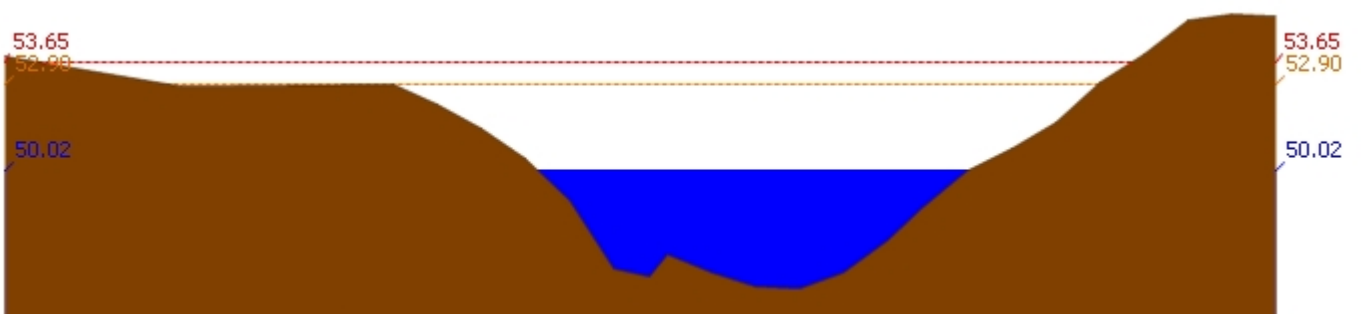
สถานี 120113T แม่น้ำป่าสักที่บ้านเขาค้าง ต.คลองกระจิง อ.ศรีเทพ จ.เพชรบูรณ์ ระดับน้ำ 50.02 ม.รทก.
