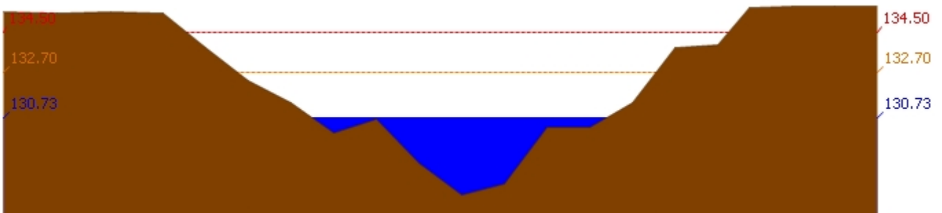
สถานี 120111T แม่น้ำป่าสักที่บ้านจางวาง ต.ลานบัว อ.หล่มสัก จ.เพชรบูรณ์ ระดับน้ำ 130.73 ม.รทก.
