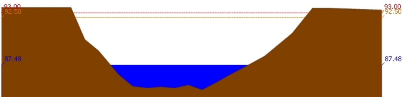
สถานี 120110T แม่น้ำป่าสักที่บ้านวังโบสถ์ ต.วังโบสถ์ อ.หนองไผ่ จ.เพชรบูรณ์ ระดับน้ำ 87.48 ม.รทก.
