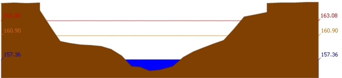
สถานี 120105T แม่น้ำป่าสักที่บ้านวังมเสหนือ ต.ทำอัญญ อ.หล่มสัก จ.เพชรบูรณ์ ระดับน้ำ 157.36 ม.รทก.
