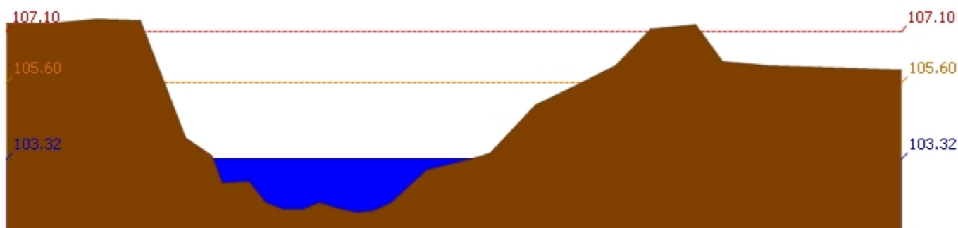
สถานี 110402T ห้วยทับเสลาที่บ้านนาไร่เดียว ต.ลานสัก อ.ลานสัก จ.อุทัยธานี ระดับน้ำ 103.32 ม.รทก.
