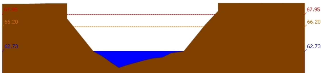
สถานี 110501T น้ำแม่วงศ์ที่บ้านคลองสาเลี ต.ลาดยาว อ.ลาดยาว จ.นครสวรรค์ ระดับน้ำ 62.73 ม.รทก.
