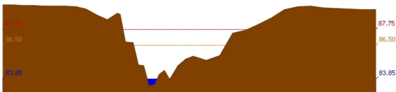
สถานี 110403T ห้วยทับเสลาที่บ้านดินแดง ต.ประดู่ยืน อ.ลานสัก จ.อุทัยธานี ระดับน้ำ 83.85 ม.รทก.
