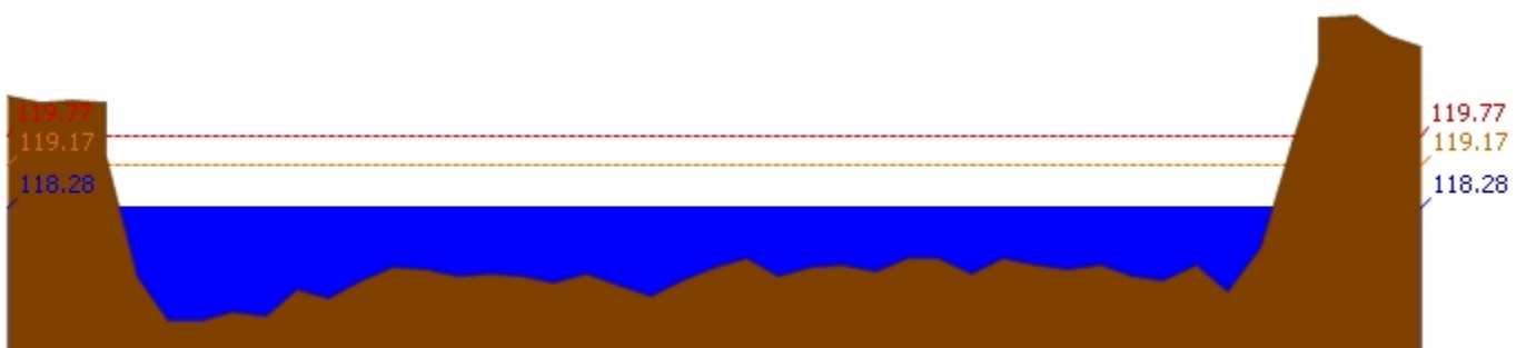
สถานี 060111T แม่น้ำปิงที่บ้านปากโรงห้วยจี้ ต.ตากออก อ.บ้านตาก จ.ตาก ระดับน้ำ 118.28 ม.รทก.
