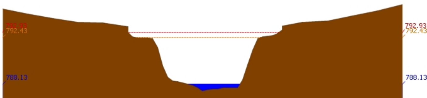
สถานี 061503T น้ำแม่ต้นที่บ้านคอย ต.ยางเปียง อ.อมก๋อย จ.เชียงใหม่ ระดับน้ำ 788.13 ม.รทก.
