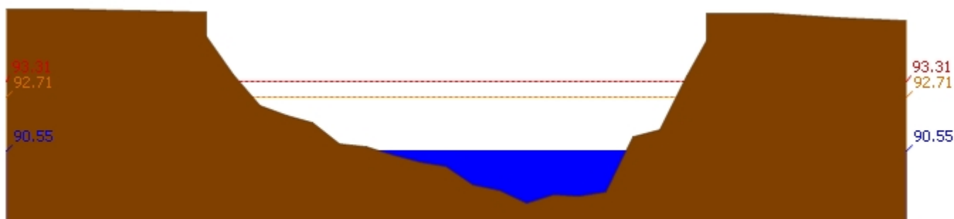
สถานี 061901T คลองแม่ระกาที่บ้านวังชะโอน ต.ท่าไม้ อ.พรานกระต่าย จ.กำแพงเพชร ระดับน้ำ 90.55 ม.รทก.
