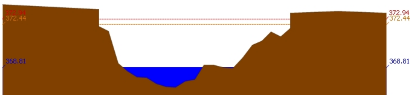
สถานี 060109T แม่น้ำปิงที่บ้านสบฮ้อ ต.แม่ระ อ.เชียงดาว จ.เชียงใหม่ ระดับน้ำ 368.81 ม.รทก.
