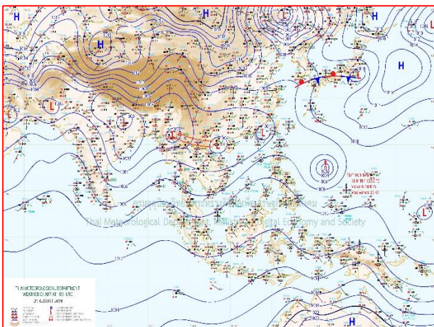
แผนที่อากาศ วันที่ ๒๑ ส.ค. ๒๕๖๒ เวลา ๐๗.๐๐ น.
