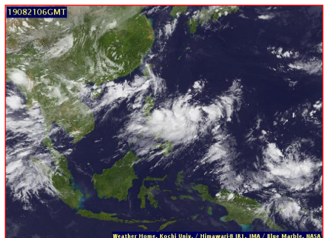
ภาพถ่ายดาวเทียม วันที่ ๒๑ ส.ค. ๒๕๖๒ เวลา ๑๓.๐๐ น.
