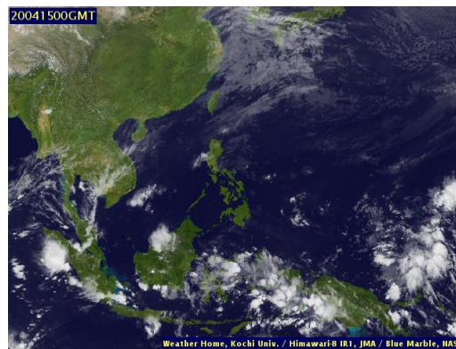
ภาพถ่ายจากดาวเทียม วันที่ 15 เม.ย. 2563
