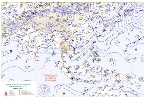
แผนที่อากาศ วันที่ 15 เม.ย. 2563 เวลา 01.00 น.
