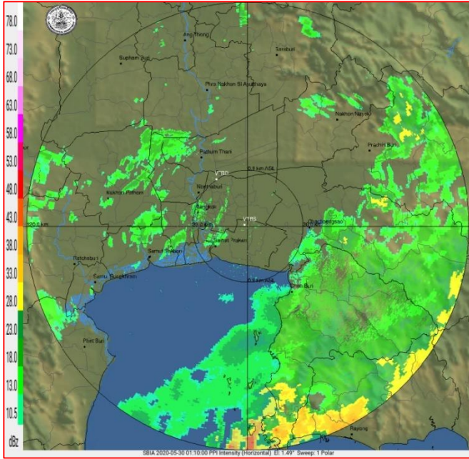
สถานีสุวรรณภูมิ เวลา ๐๘.๑๐ น.
