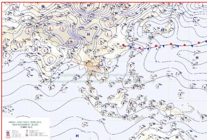
แผนที่อากาศ วันที่ ๓๐ พ.ค. ๒๕๖๓ เวลา ๐๑.๐๐ น.
