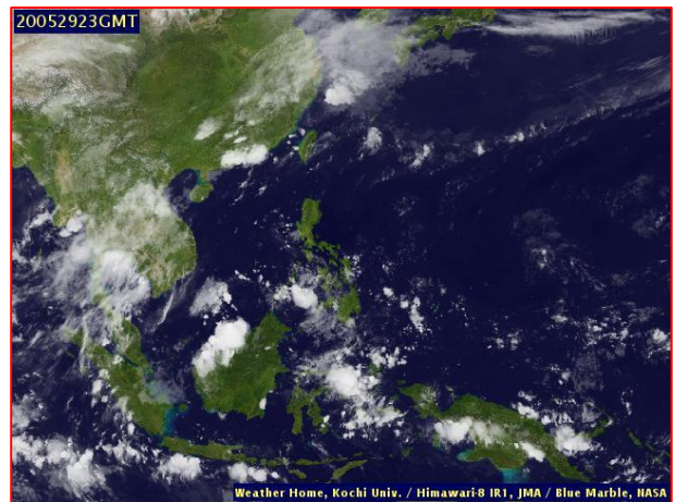
ภาพถ่ายดาวเทียม วันที่ ๓๐ พ.ค. ๒๕๖๓ เวลา ๐๖.๐๐ น.
