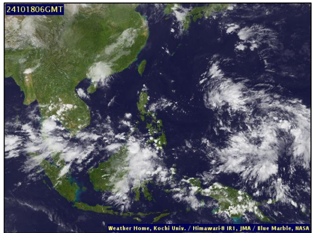
ภาพถ่ายดาวเทียม วันที่ ๑๘ ต.ค. ๒๕๖๗ เวลา ๑๓.๐๐ น.
