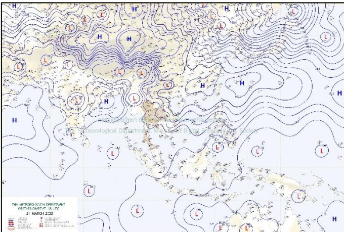
แผนที่อากาศ วันที่ ๒๒ มี.ค. ๒๕๖๘ เวลา ๐๑.๐๐ น.
