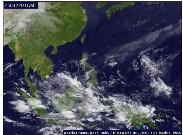
ภาพถ่ายดาวเทียม วันที่ ๒๒ มี.ค. ๒๕๖๘ เวลา ๐๘.๐๐ น.
