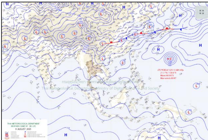
แผนที่อากาศ วันที่ ๑๐ ส.ค. ๒๕๖๘ เวลา ๐๑.๐๐ น.
