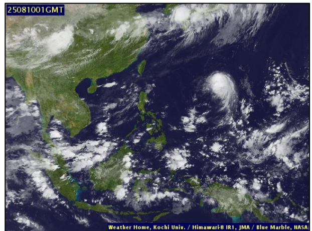
ภาพถ่ายดาวเทียม วันที่ ๑๐ ส.ค. ๒๕๖๘ เวลา ๐๘.๐๐ น.
