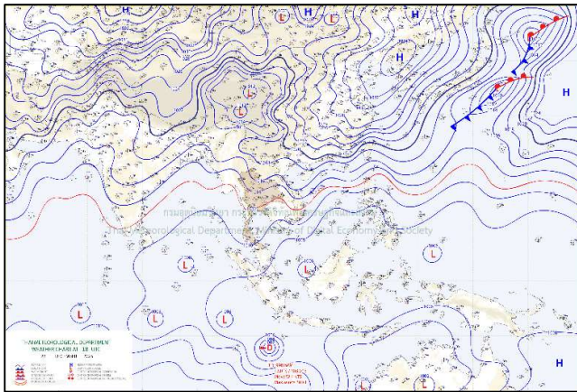
แผนที่อากาศ วันที่ ๒๒ ธ.ค. ๒๕๖๘ เวลา ๐๑.๐๐ น.
