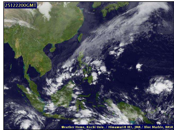
ภาพถ่ายดาวเทียม วันที่ ๒๒ ธ.ค. ๒๕๖๘ เวลา ๐๗.๐๐ น.
