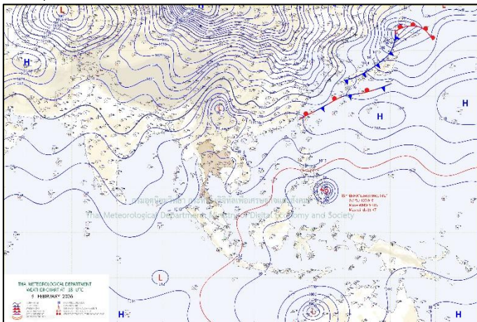
แผนที่อากาศ วันที่ ๖ ก.พ. ๒๕๖๙ เวลา ๐๑.๐๐ น.
