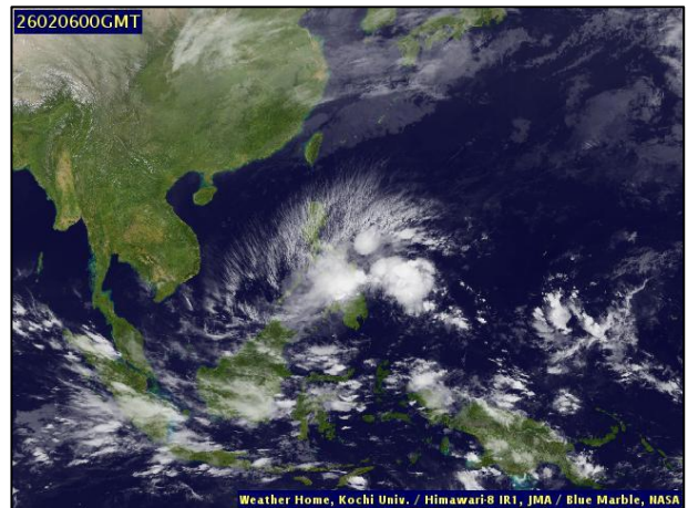
ภาพถ่ายดาวเทียม วันที่ ๖ ก.พ. ๒๕๖๙ เวลา ๐๗.๐๐ น.
