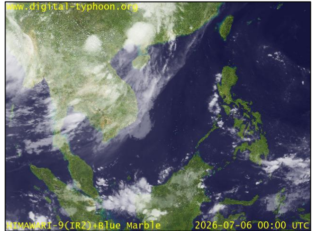
ภาพถ่ายดาวเทียม วันที่ ๖ ก.ค. ๒๕๖๙ เวลา ๐๗.๐๐ น.
