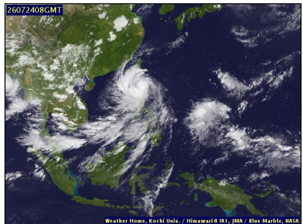
ภาพถ่ายดาวเทียม วันที่ ๒๔ ก.ค. ๒๕๖๙ เวลา ๑๕.๐๐ น.
