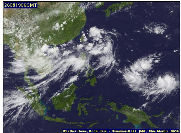
ภาพถ่ายดาวเทียม วันที่ ๑๙ ส.ค. ๒๕๖๙ เวลา ๑๓.๐๐ น.
