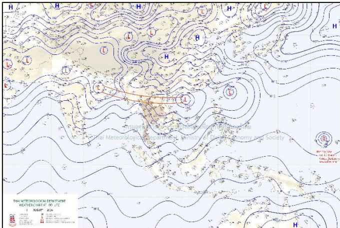
แผนที่อากาศ วันที่ ๑๙ ส.ค. ๒๕๖๙ เวลา ๐๗.๐๐ น.
